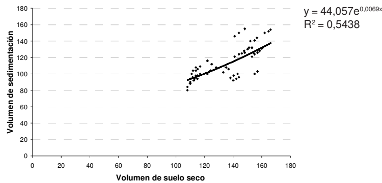
Figura 4. Modelo exponencial
