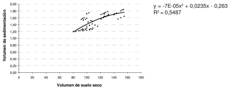
Figura 3. Modelo cuadrático
