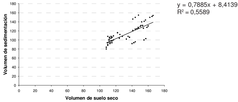
Figura 2. Modelo lineal
