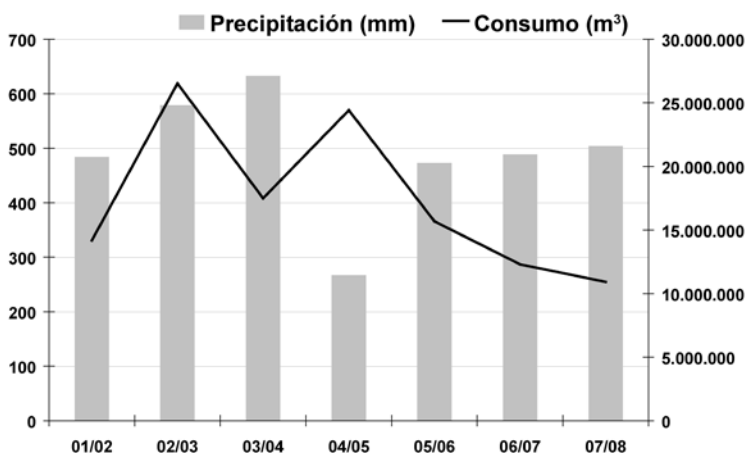
Figura 3. Evolución anual de la precipitación y de los consumos totales. Figure 3. Annual evolution of precipitation and total water consumptions.
