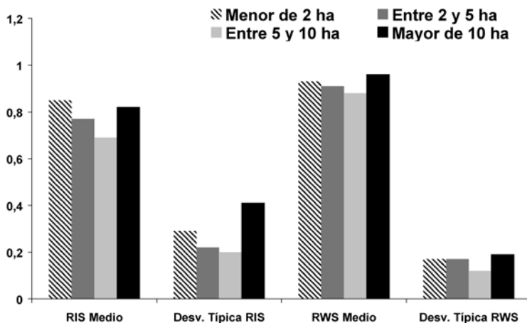
Figura 11. Comparación del valor medio y desviación típica de los indicadores RIS y RWS según tamaño de la parcela.
