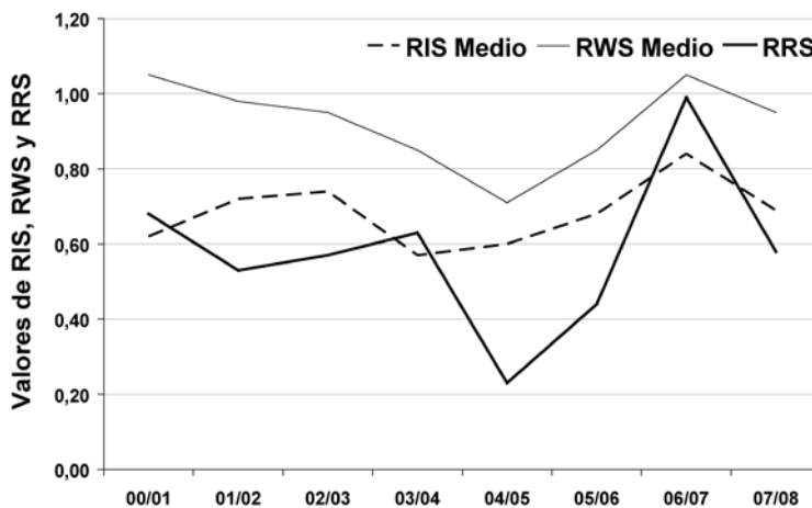
Figura 8. Evolución de los indicadores para un suelo de textura franco arcillo limosa. Figure 8. Evolution of indicators in a silty clay loam texture soil.
