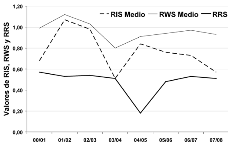
Figura 6. Evolución de los indicadores en riego por aspersión.
