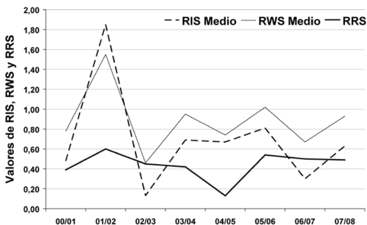
Figura 9. Evolución de los indicadores para un suelo de textura franco arenosa. Figure 9. Evolution of indicators in a sandy loam texture soil.
