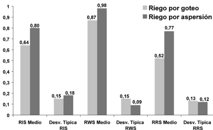
Figura 7. Comparación del valor medio y desviación típica de los indicadores según el tipo de riego.
