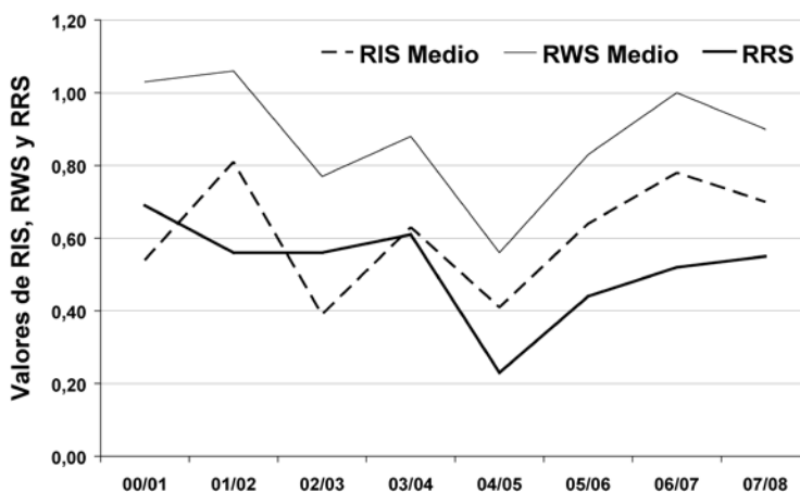
Figura 5. Evolución de los indicadores en riego por goteo.
